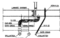
PRINCIPSEKTION ANSL. AV VÄRMELEDNING TILL SÄMNINGSDIVISION 1 ÖRIND SKALA 1:20
