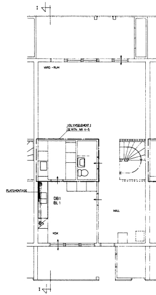
BOTTENPLAN SKALA 1:50
