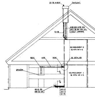
SEKTION I-I SKALA 1:50
